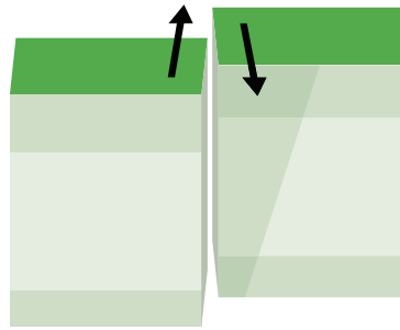
FAILLE DÉCROCHANTE
